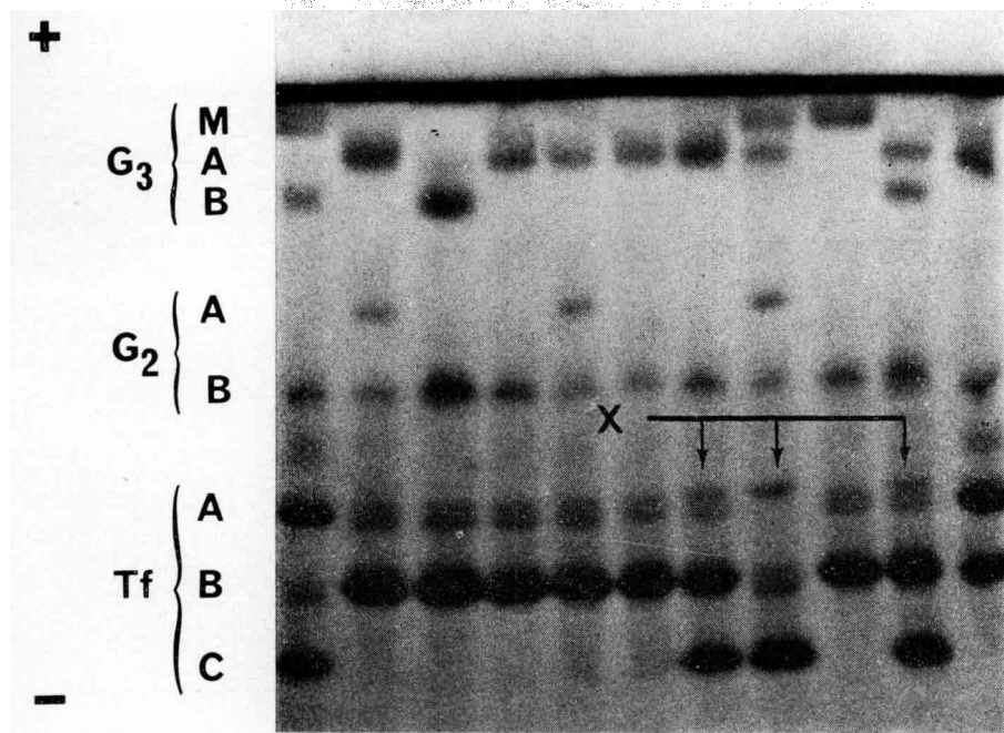
FIG. 1. — Protéinogramme d'albumen de diverses formules génétiques Les lettres M, A, B et C de la partie gauche de l'illustration désignent les différentes formes ou variants génétiques de l'ovoglobuline G_3(G_3) , de l'ovoglobuline G_2(G_2) et de la conalbumine (Tf). Les zones fléchées sur la photographie correspondent au constituant X associé au variant C de la conalbumine.
