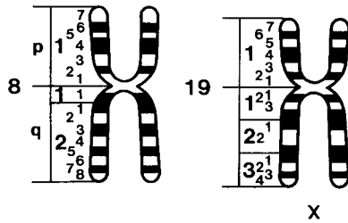
FIG. 2. — Diagrammatic representation of the bands and landmarks on chromosome No. 8 and the X chromosome of the domestic pig Représentation schématique des bandes et des landmarks du chromosome X et du chromosome 8 du Porc domestique
